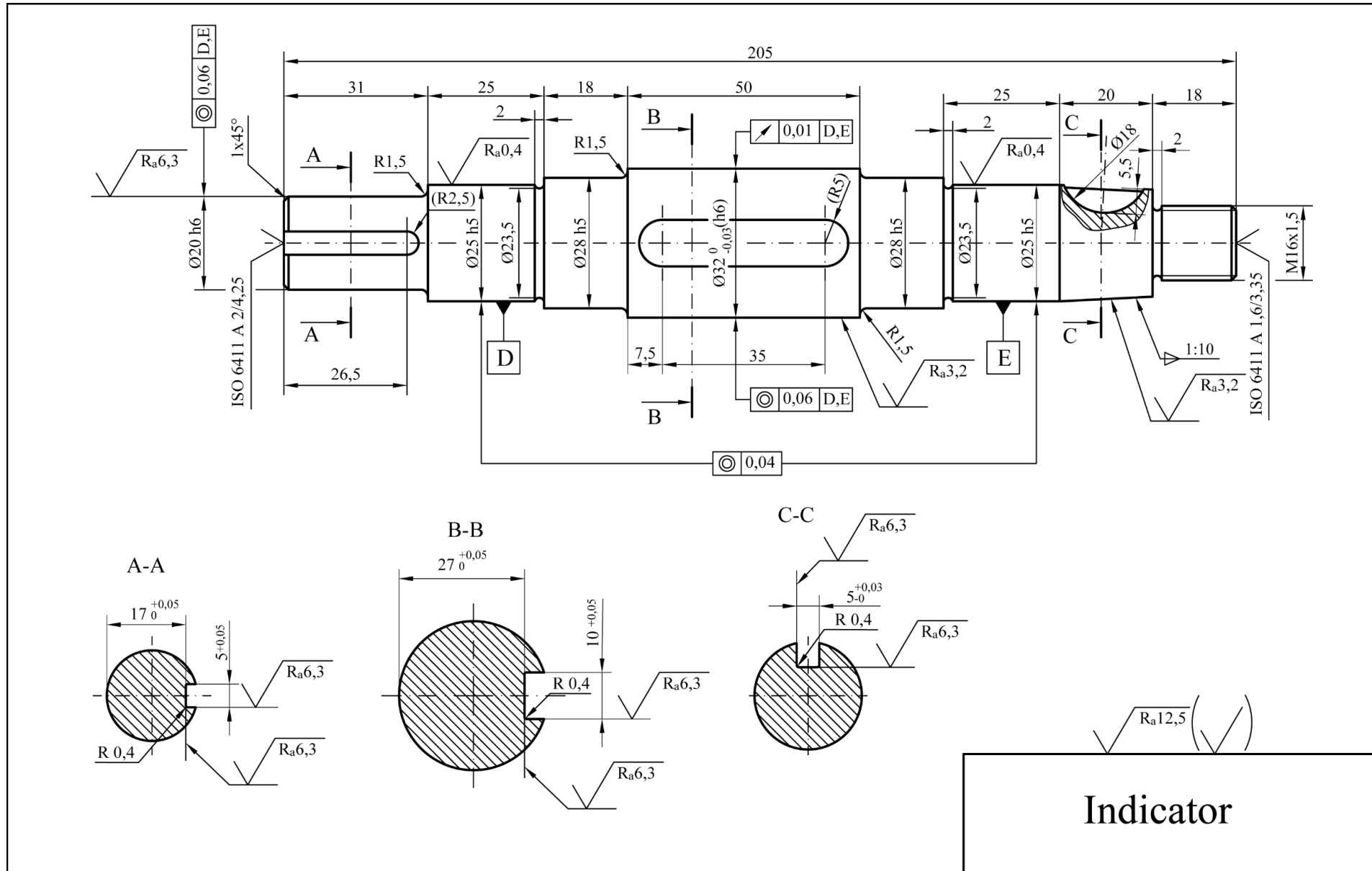
Desen de execuție arbore drept
