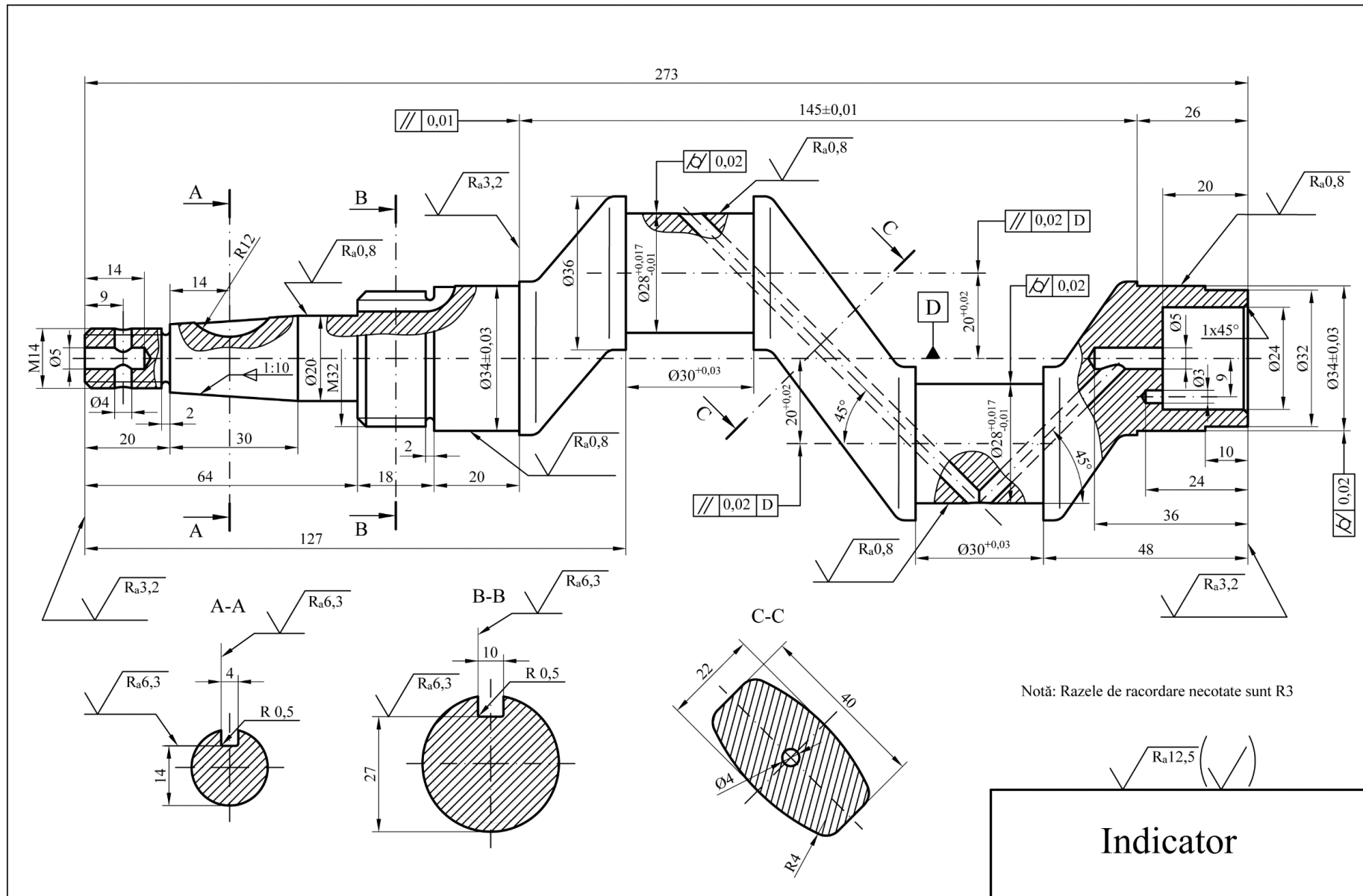
Desen de execuție arbore cotit
